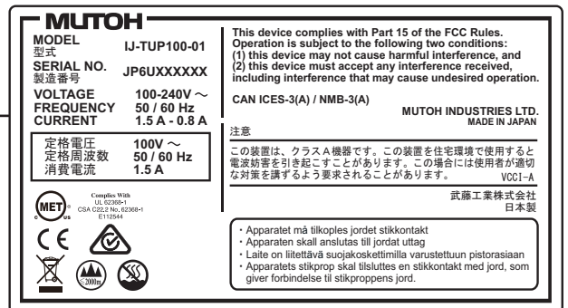
定格銘版
